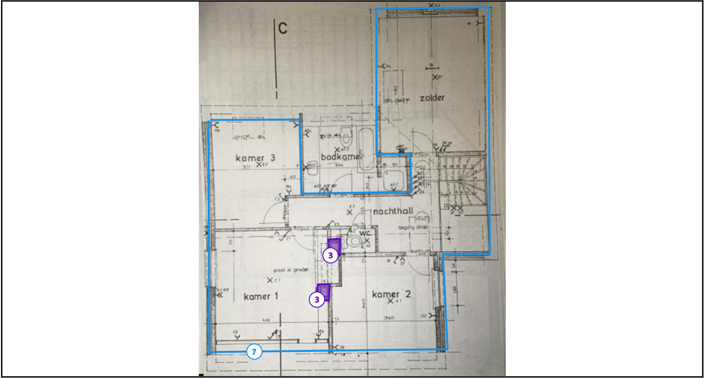
Legende van plan 1.4: Plan - 1ste verdieping
